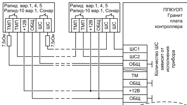
Рис.Б3 Схема подключения охранных извещателей Рapid вар.1,4,5, Рapid-10 вар.1, Сонар (тампер подключён к отдельному ШС)
